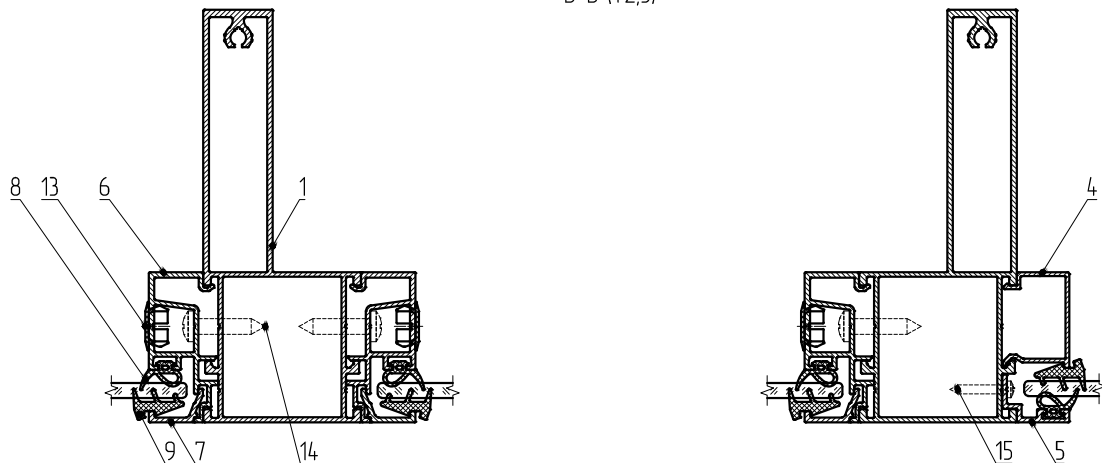
В-В (1:2,5)
