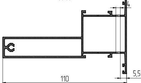
Д-Д
