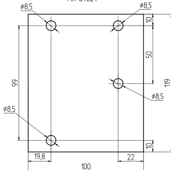
Мех. обработка шины 100х5-DIN(C) L=119 мм для крепления стоек МП-64024
