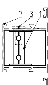
Сечение по створке (открывание наружу)
