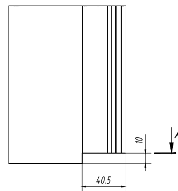
Вид А Мехобработка низа стойки
