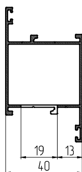
Г-Г
