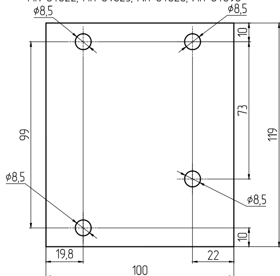
Мех. обработка шины 100х5-DIN(C) L=119 мм для крепления стоек МП-64022, МП-64023, МП-64028, МП-64090
