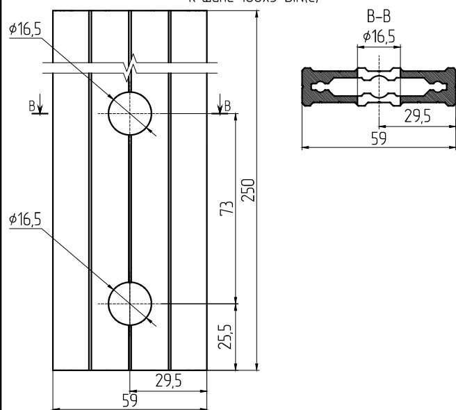
B-B
