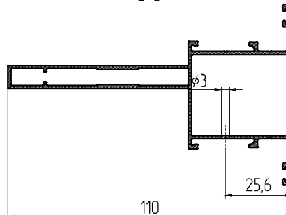
Б-Б
